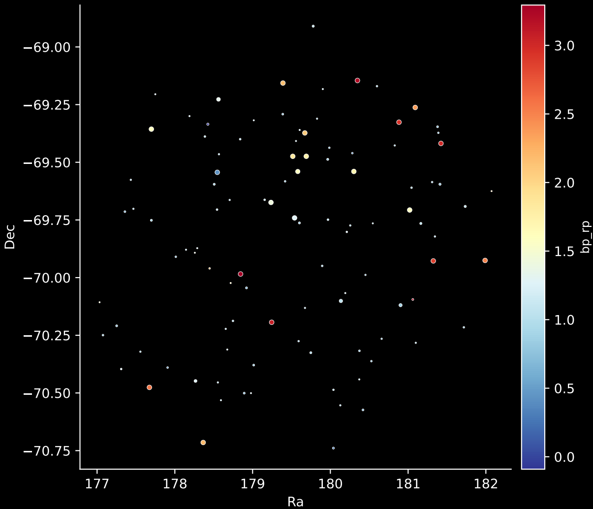
APOGEE DR17 Field: [281-33-O_TESS] Stars: 104
