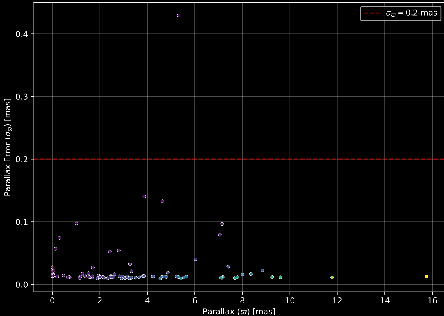
APOGEE DR17 Field: [281-33-O_TESS] Parallax Quality (n= 104)
