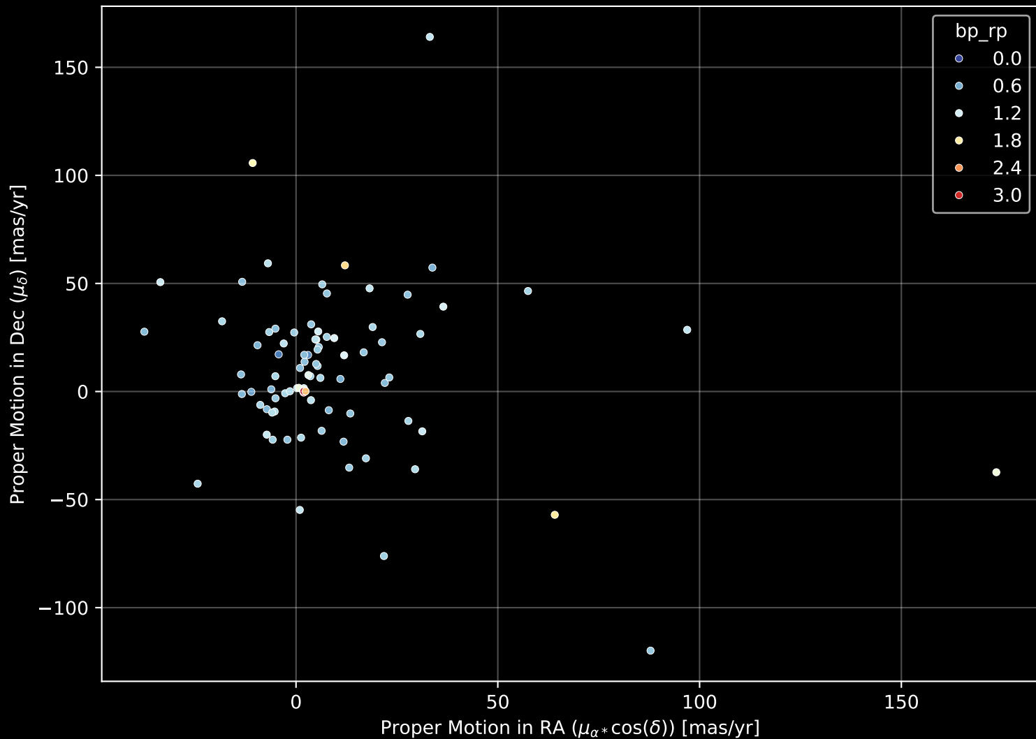
APOGEE DR17 Field: [281-33-O_TESS] Proper Motion Diagram (n= 104)
