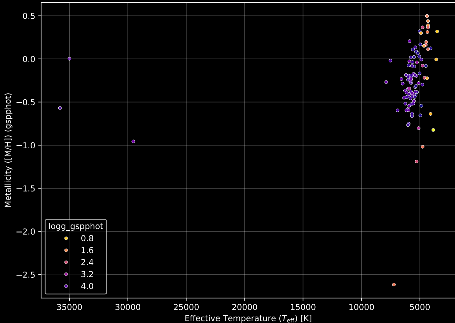
APOGEE DR17 Field: [281-33-O_TESS] Stellar Population Parameters (n= 104)
