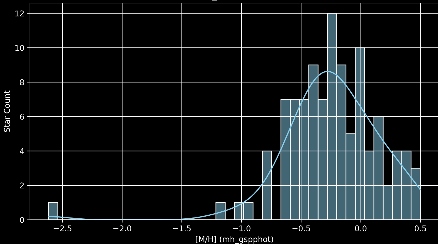
APOGEE DR17 Field: [281-33-O_TESS [M/H] (mh_gspphot) (n= 104)
